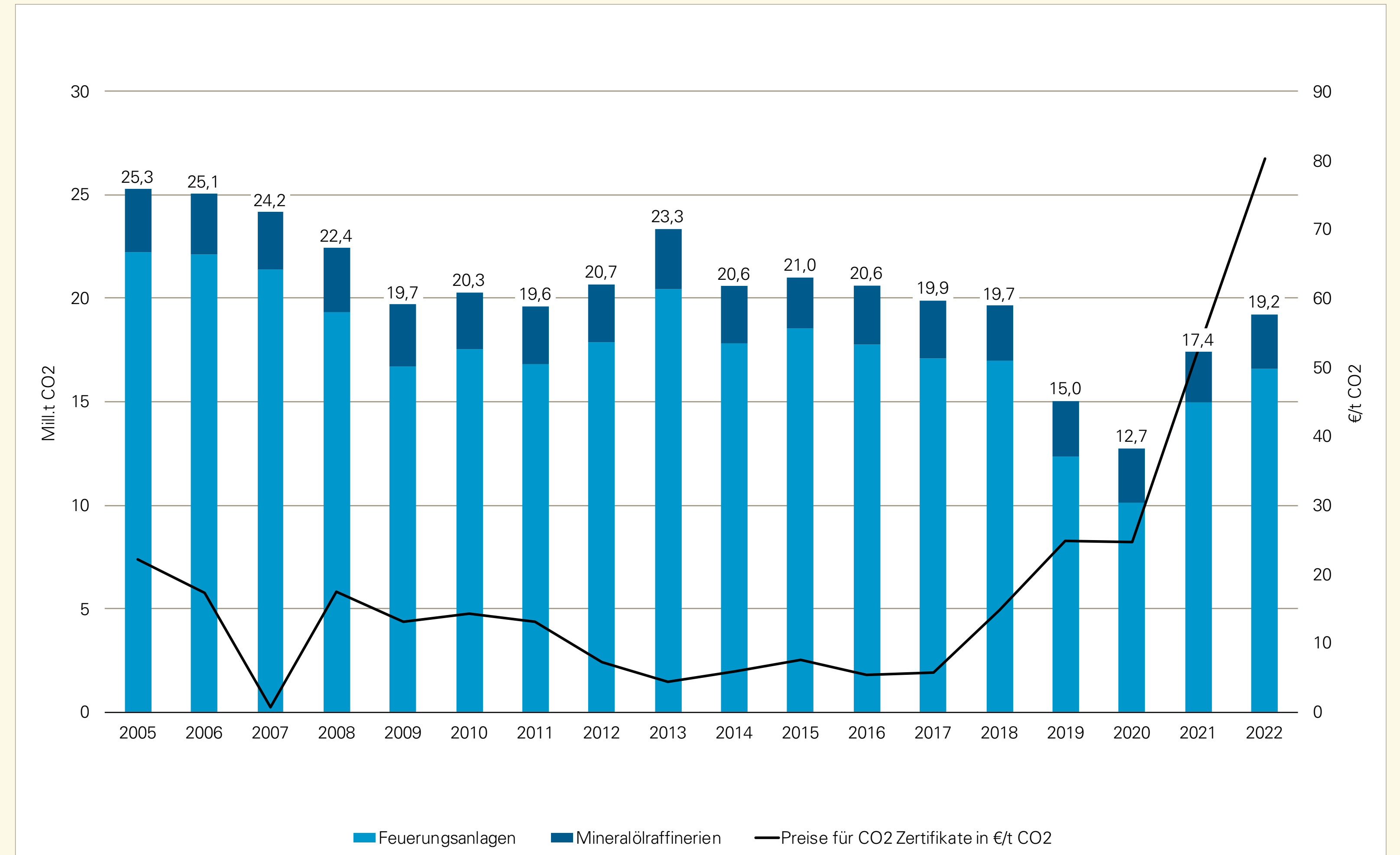
ABBILDUNG 4: ENTWICKLUNG DER CO 2 -EMISSIONEN DER ENERGIEANLAGEN (STROM-, FERNWÄRME- UND PROZESSWÄRMEERZEUGUNG) UND MINERALÖLRAFFINERIEEN IM RAHMEN DES ETS IN BADEN-WÜRTTEMBERG VON 2005 BIS 2022
