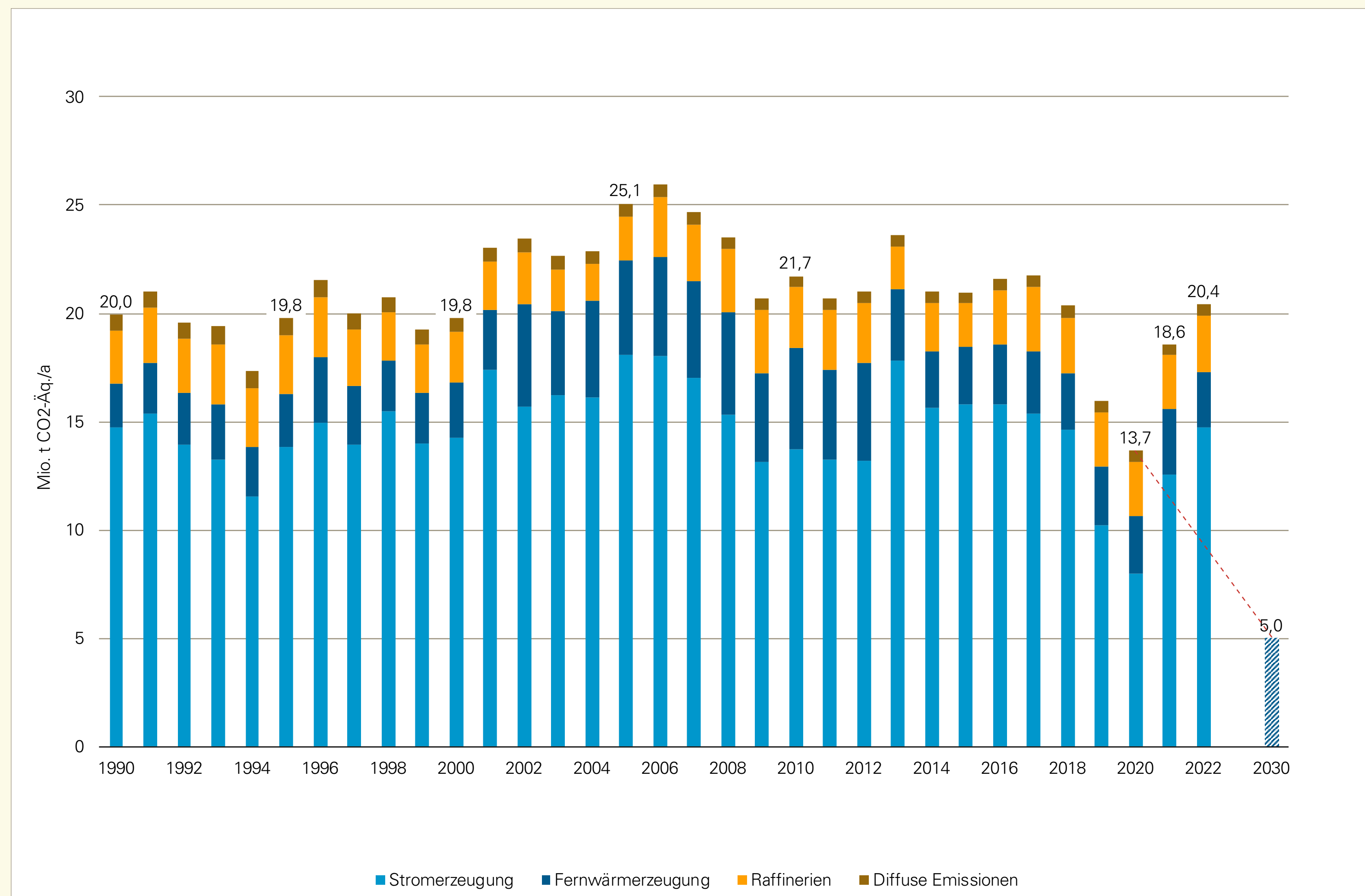
ABBILDUNG 6: ENTWICKLUNG DER TREIBHAUSGASEMISSIONEN DER ENERGIEWIRTSCHAFT IN BADEN-WÜRTTEMBERG VON 1990 BIS 2021
