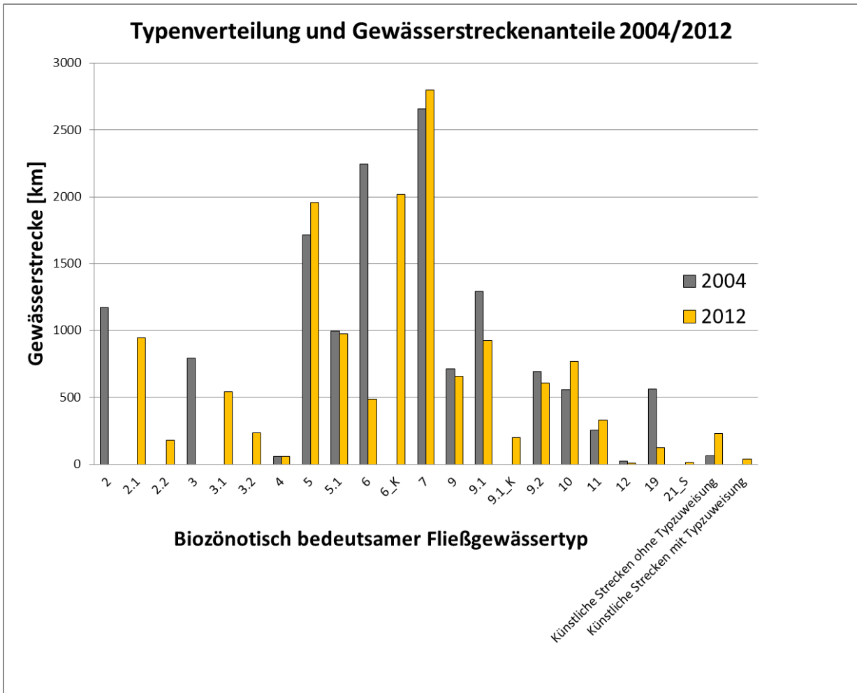
Abb.8: Streckenmäßige Verteilung der Fließgewässertypen in Baden-Württemberg vor der Überprüfung (2004) und nach der Überprüfung (2012)
