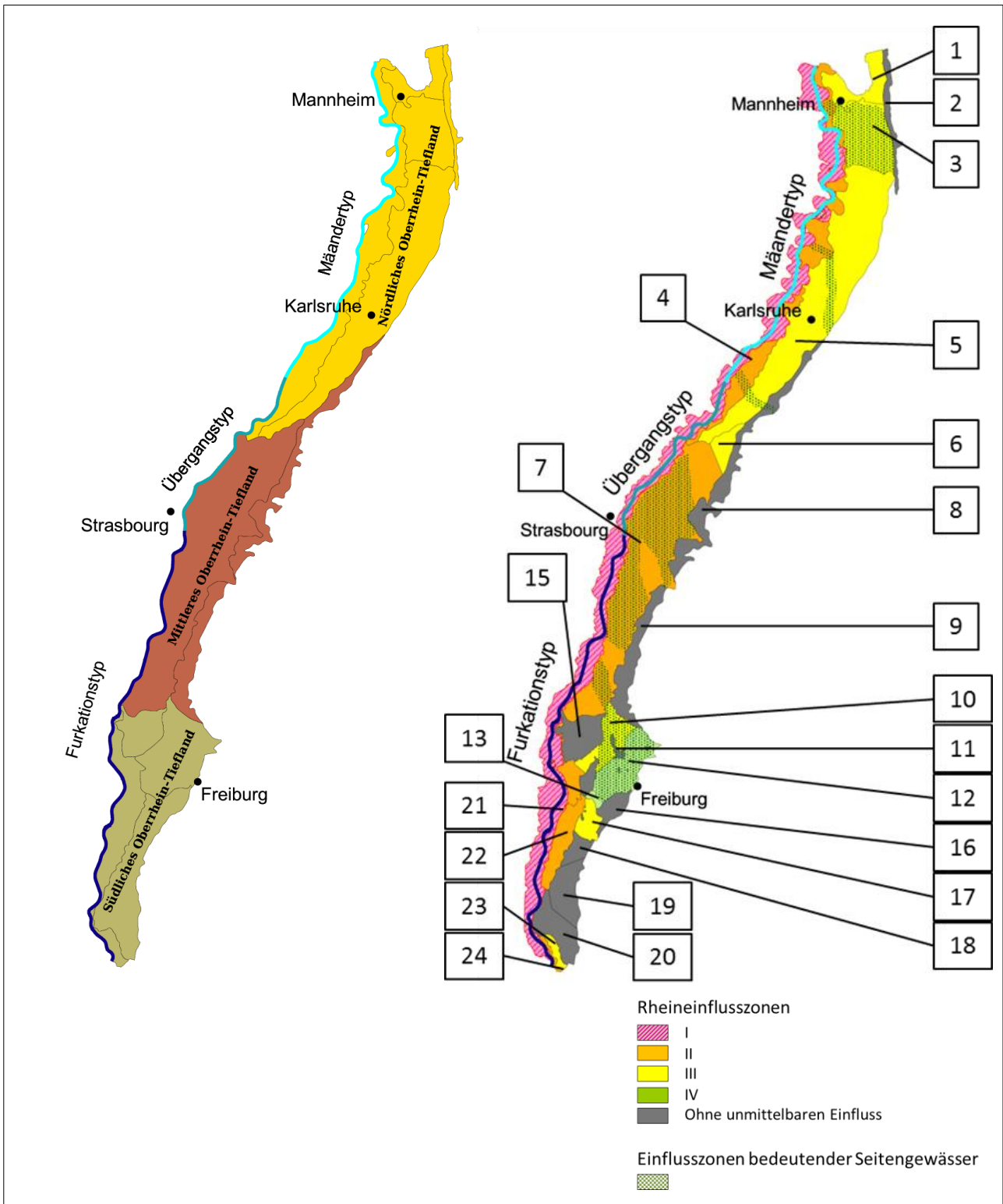
Abb.5: Links: Naturräumliche Gliederung BW, rechts: feinere Untergliederung im Rahmen des Konzeptes zur Typisierung der Fließgewässer in der Oberrheinebene
