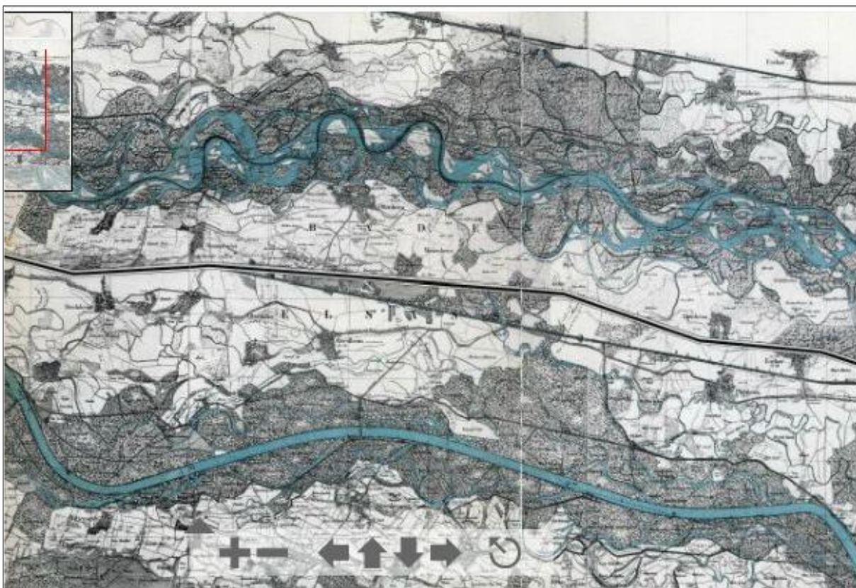
Abb.7: Längerer Ausschnitt aus dem Rheinlauf von Weisweil bis Marlen, oberer Teil um 1828 (vor der „Rheinkorrektur“) unterer Teil um 1882 (nach der Rheinkorrektur)
