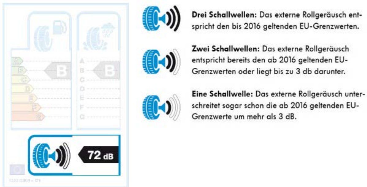
Abb. 3: Angabe des externen Rollgeräusches gemäß Europäischer Reifen-Kennzeichnungs-Verordnung 1222/2009
