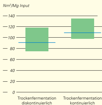
ABB. 25: GASERTRÄGE BEI DER TROCKENFERMENTATION VON BIOABFÄLLEN (WI & PÖYRY 2009)
