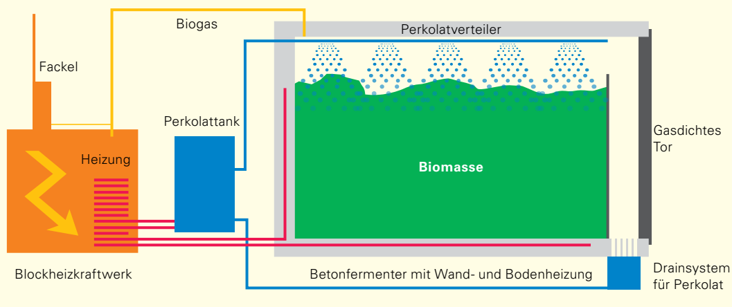
ABB. 24: BEISPIELHAFTES VERFAHRENSSCHEMA EINER DISKONTINUIERLICHEN TROCKENVERGÄRUNG IN BOXENFERMENTERN (QUELLE: FA. BEKON)
