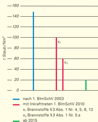
ABB.18: ENTWICKLUNG DER GRENZWERTE FÜR STAUBEMIS- SIONEN GEMÄSS DER 1. BlmSchV FÜR NEU ERRICHTETE WÄRME- ERZEUGUNGSANLAGEN FÜR FESTE BRENNSTOFFE MIT EINER FEUERUNGSWÄRMELEISTUNG BIS 1 MW
