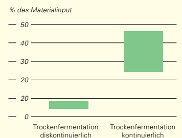
ABB. 26: ÜBERSCHUSSWASSER BEI DER TROCKENFERMENTATION VON BIOABFÄLLEN (WI & PÖRY 2009)
