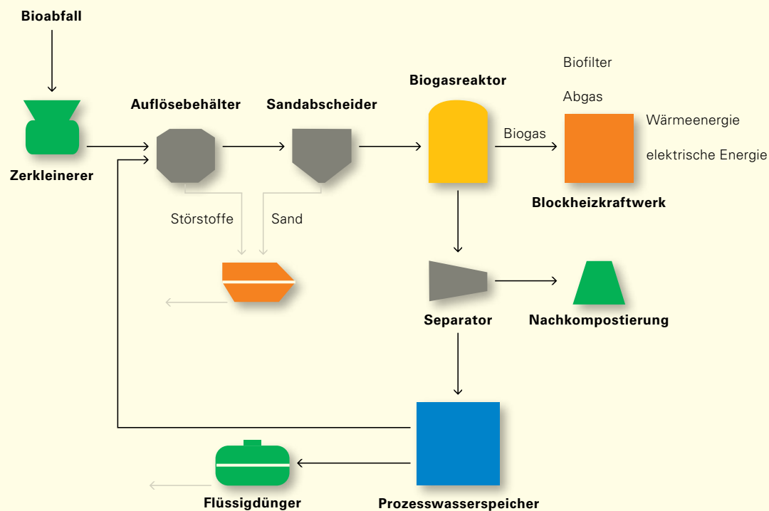
ABB. 22: BEISPIELHAFTES VERFAHRENSSCHEMA DER KONTINUIERLICHEN NASSVERGÄRUNG VON BIOABFÄLLEN (QUELLE: FA. BTA)
