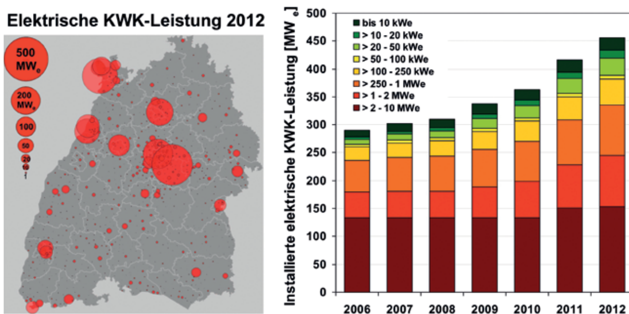
Abbildung 2: Räumliche Verteilung der KWK-Leistung (inkl. Anlagen > 10 MW e ) in 2012 sowie Entwicklung der Kraftwerksleistung in Kraft-Wärme-Kopplungs-Anlagen (< 10 MW e ) in Baden-Württemberg von 2006 bis 2012. Quelle: BAFA 2013
