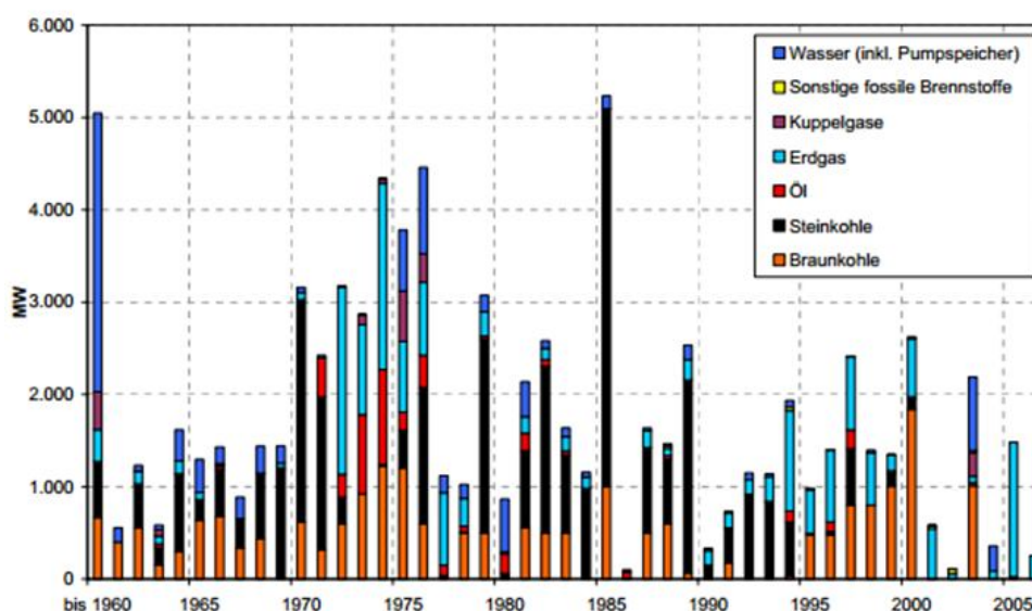
Abbildung 4: Inbetriebnahme von Kraftwerkskapazitäten zwischen 1960 und 2005
