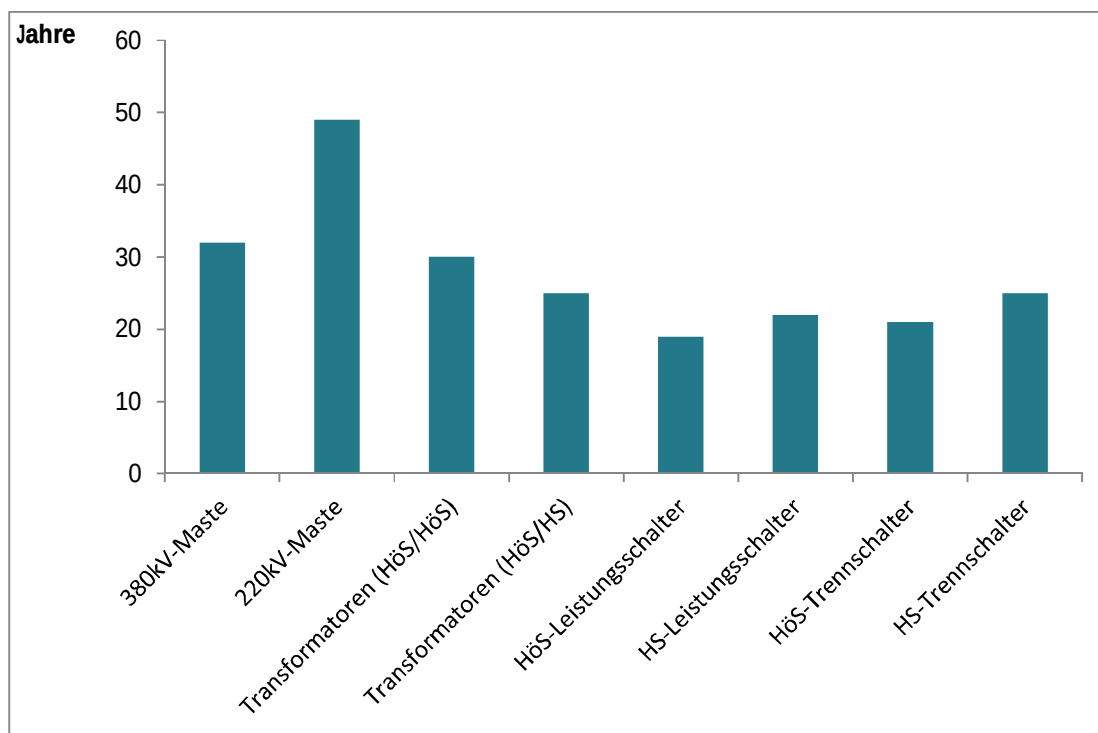
Abbildung 7: Durchschnittsalter diverser Komponenten im deutschen Höchstspannungsnetz
