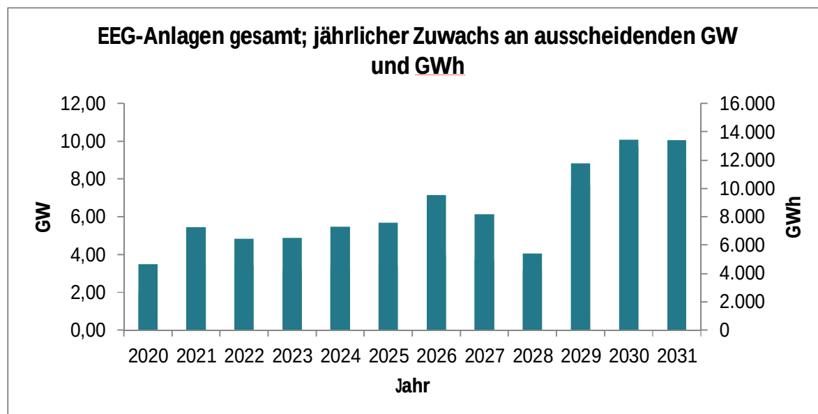
Abbildung 5: Leistung und voraussichtliche Arbeit aus Anlagen, die nach 2020 aus dem EEG herausfallen, ohne Berücksichtigung wahrscheinlicher Repowering-Maßnahmen
