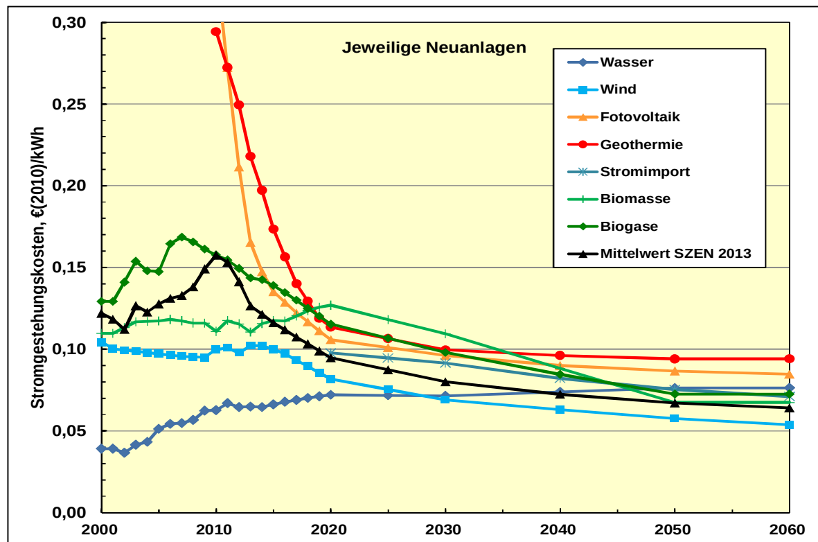
Abbildung 6: Stromgestehungskosten von EE-Neuanlagen (mit Wärmegutschriften bei Geothermie und Biomasse)
