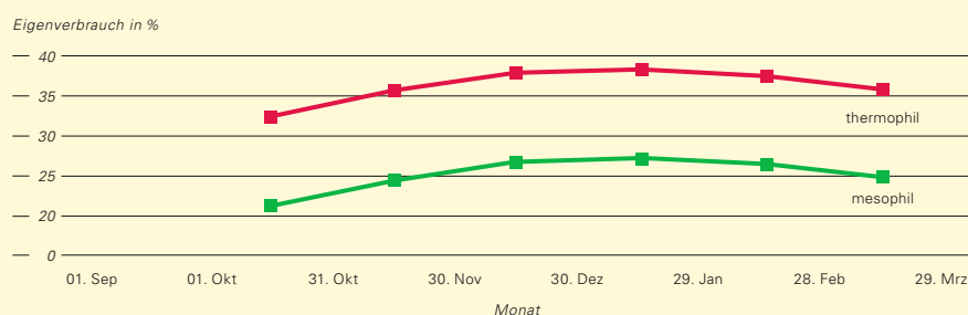
ABB. 41: EXEMPLARISCHER WÄRMEEIGENBEDARF VON VERGÄRUNGSANLAGEN IN DEN WINTERMONATEN (UBA 2010)
