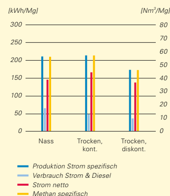
ABB. 35: STROMERZEUGUNG UND STROMBEDARF SOWIE NETTO-STROM-AUSBEUTE BEZOGEN AUF DEN ANLAGEN-INPUT BEI NASS- UND TROCKEN-VERGÄRUNGSVERFAHREN VON BIO- UND GRÜNGUT (FRICKE 2013)
