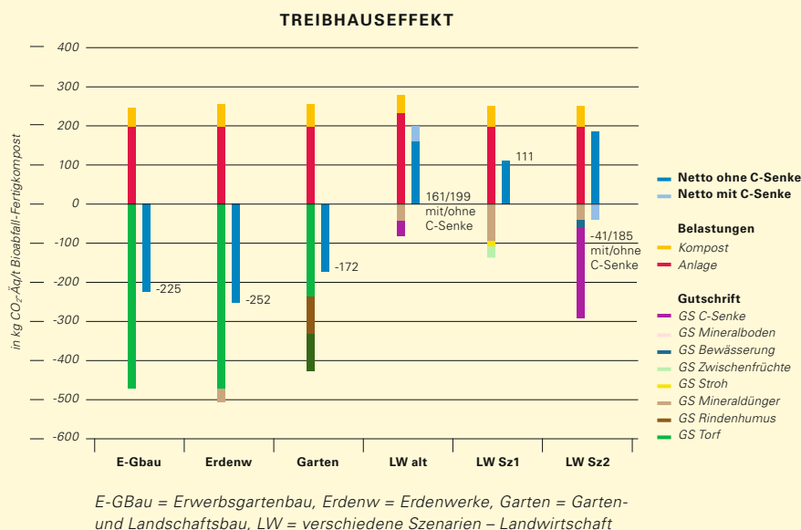
ABB. 22: VERGLEICH DER ABSATZOPTIONEN VON FERTIGKOMPOST AUS ÖKOLOGISCHER SICHT AM BEISPIEL TREIBHAUSEFFEKT (IFEU/AHU 2012)
