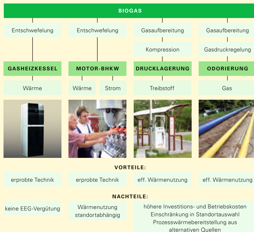
ABB. 39: ÜBERSICHT ÜBER DIE BIOGASNUTZUNGSKONZEPTE
