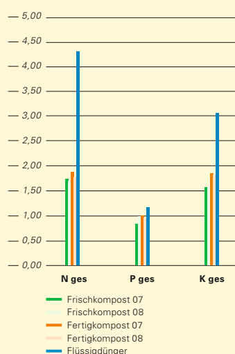
ABB. 38: VERGÄRUNG VON BIOGUT MIT ANSCHLIESSENDER FEST-FLÜSSIG-TRENNUNG DES GÄRRESTS – DARSTELLUNG DER NÄHRSTOFFGEHALTE IN PROZENT TROCKENSUBSTANZ FÜR UNTERSCHIEDLICHE MATERIALPROBEN (FRISCHKOMPOST 07 ETC. PP.) (NACH ABFALLWIRTSCHAFTSBETRIEB WETTERAUKREIS)
