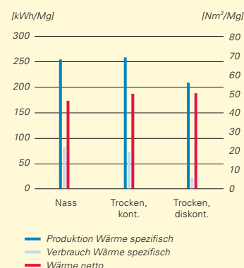
ABB. 36: WÄRMERZEUGUNG UND WÄRMEBEDARF SOWIE NETTO-WÄRMERZEUGUNG BEZOGEN AUF DEN ANLAGEN-INPUT BEI NASS- UND TROCKEN-VERGÄRUNGSVERFAHREN VON BIO- UND GRÜNGUT (FRICKE 2013)
