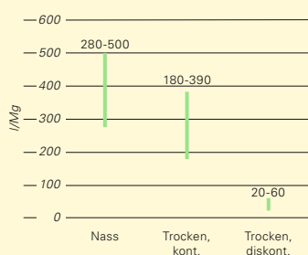
ABB. 37: ÜBERSCHUSSWASSER BEI DER VERGÄRUNG VON BIO- UND GRÜNGUT DIFFERENZIIERT NACH VERFAHRENS- UND PROZESSARTEN, BEZOGEN AUF DEN MATERIALINPUT (FRICKE 2013)
