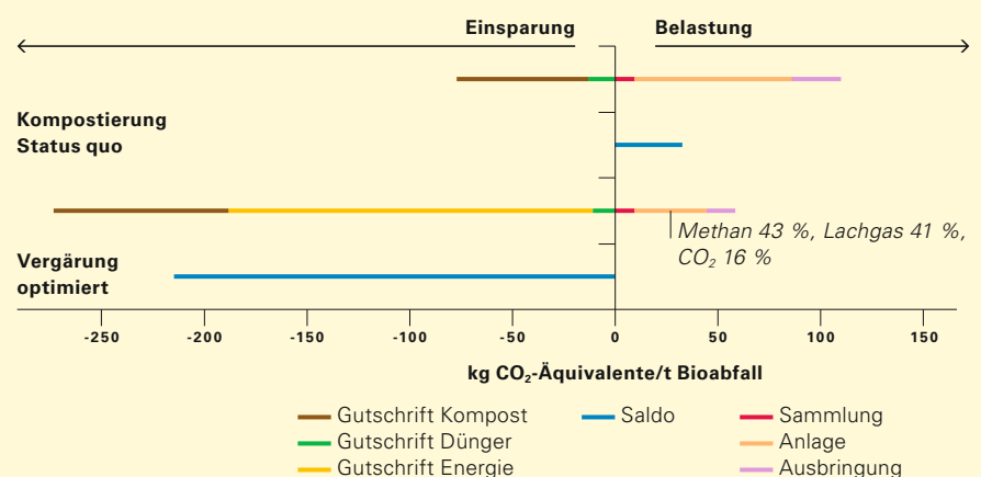
ABB. 28: ALTERNATIVE DER KOMPOSTIERUNG UND VERGÄRUNG VON BIOABFÄLLEN AUS SIGHT DES KLIMASCHUTZES (LUBW/IFEU 2010)
