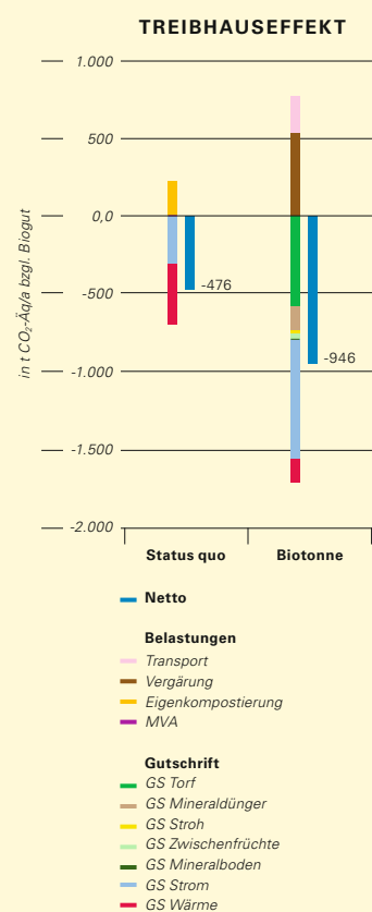
ABB. 20: EINFÜHRUNG DER BIOTONNE AUS ÖKOLOGISCHER SICHT (UNTER KLIMASPEKTEN)
